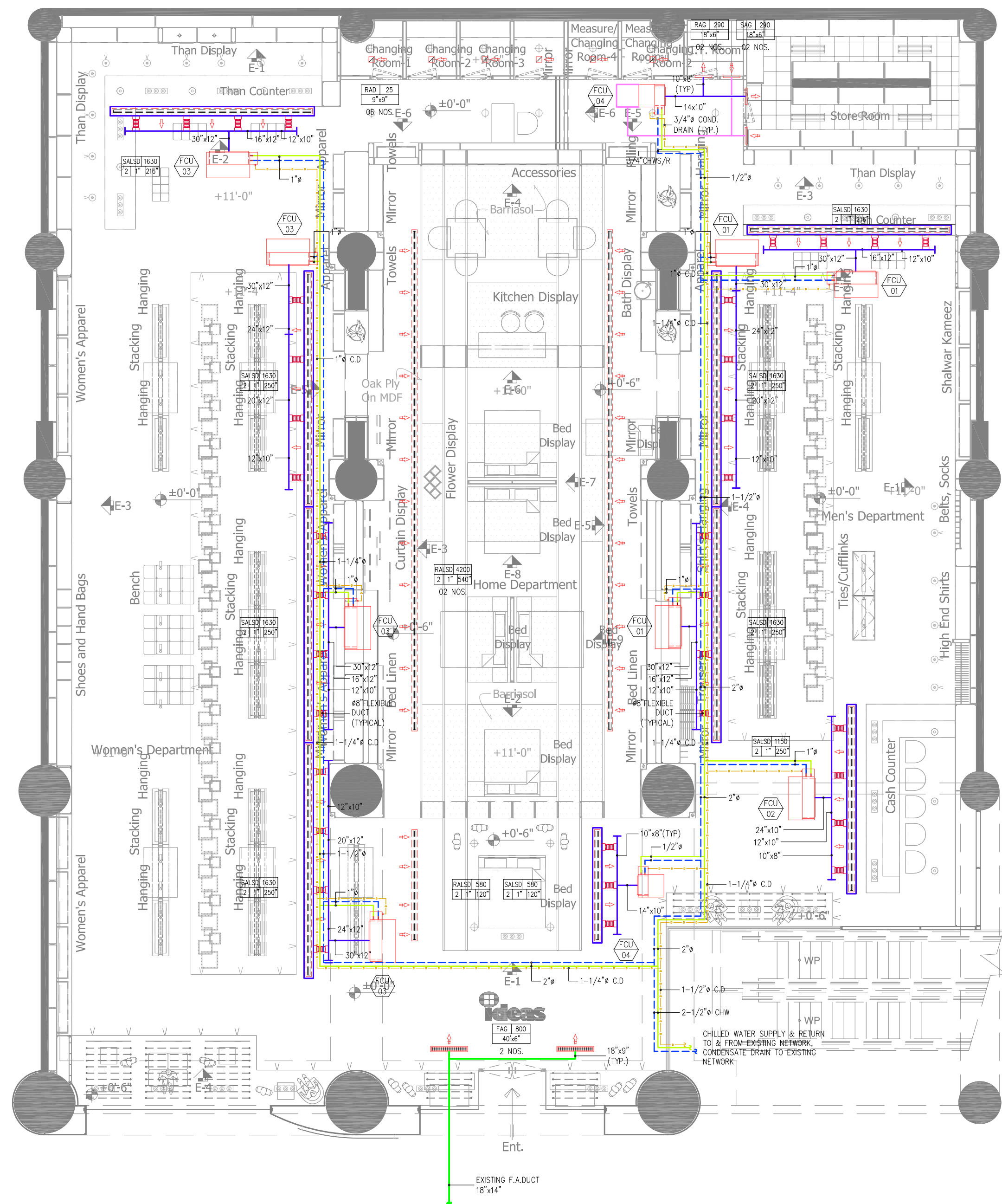
1 HVAC LAYOUT M.03 SCALE: 1/8"=1'-0"
